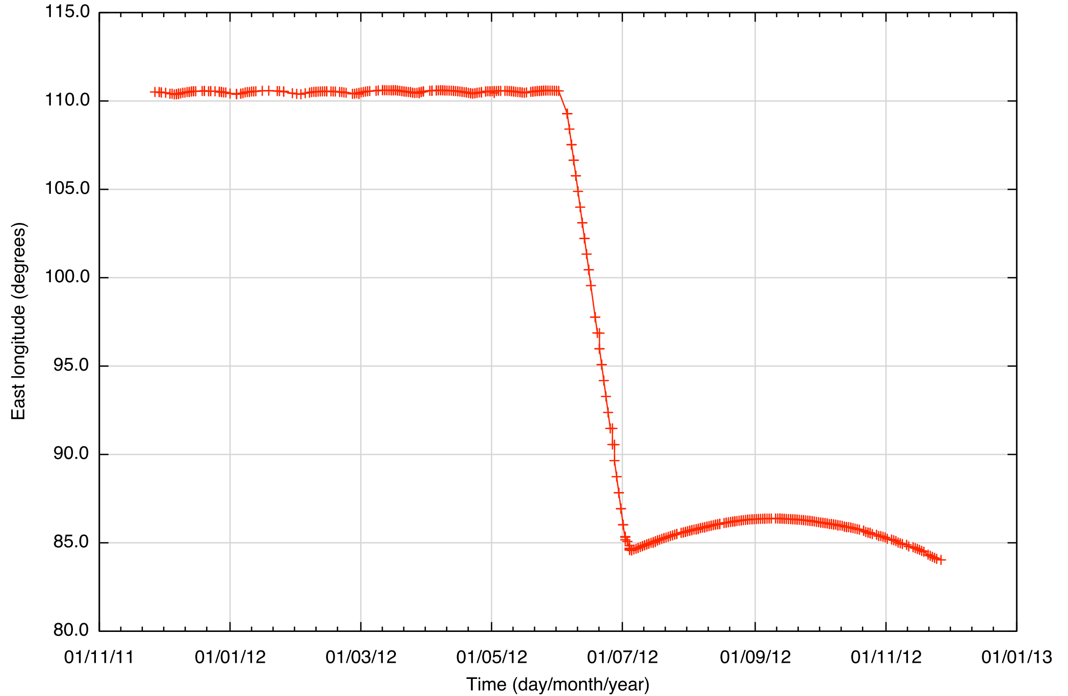
BeiDou 1C Orbit Longitude
